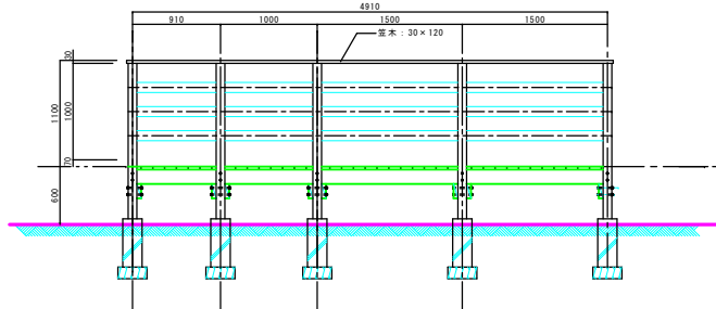
立面図
