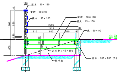
断面図
