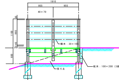
立面図
